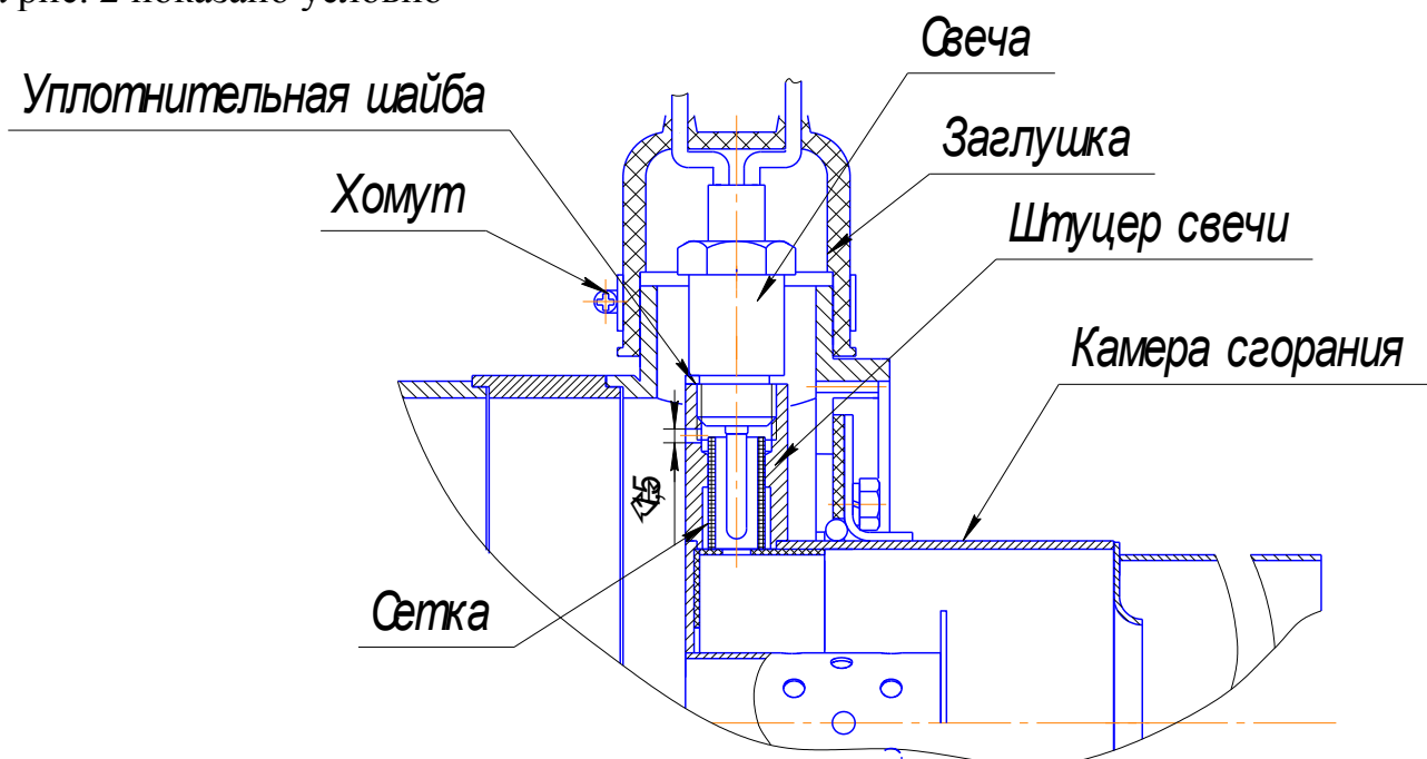
Рис 2- Схема установки втулки и сетки в камеру сгорания.
