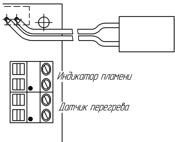
Рис.7а – Подключение (в блоке управления)
