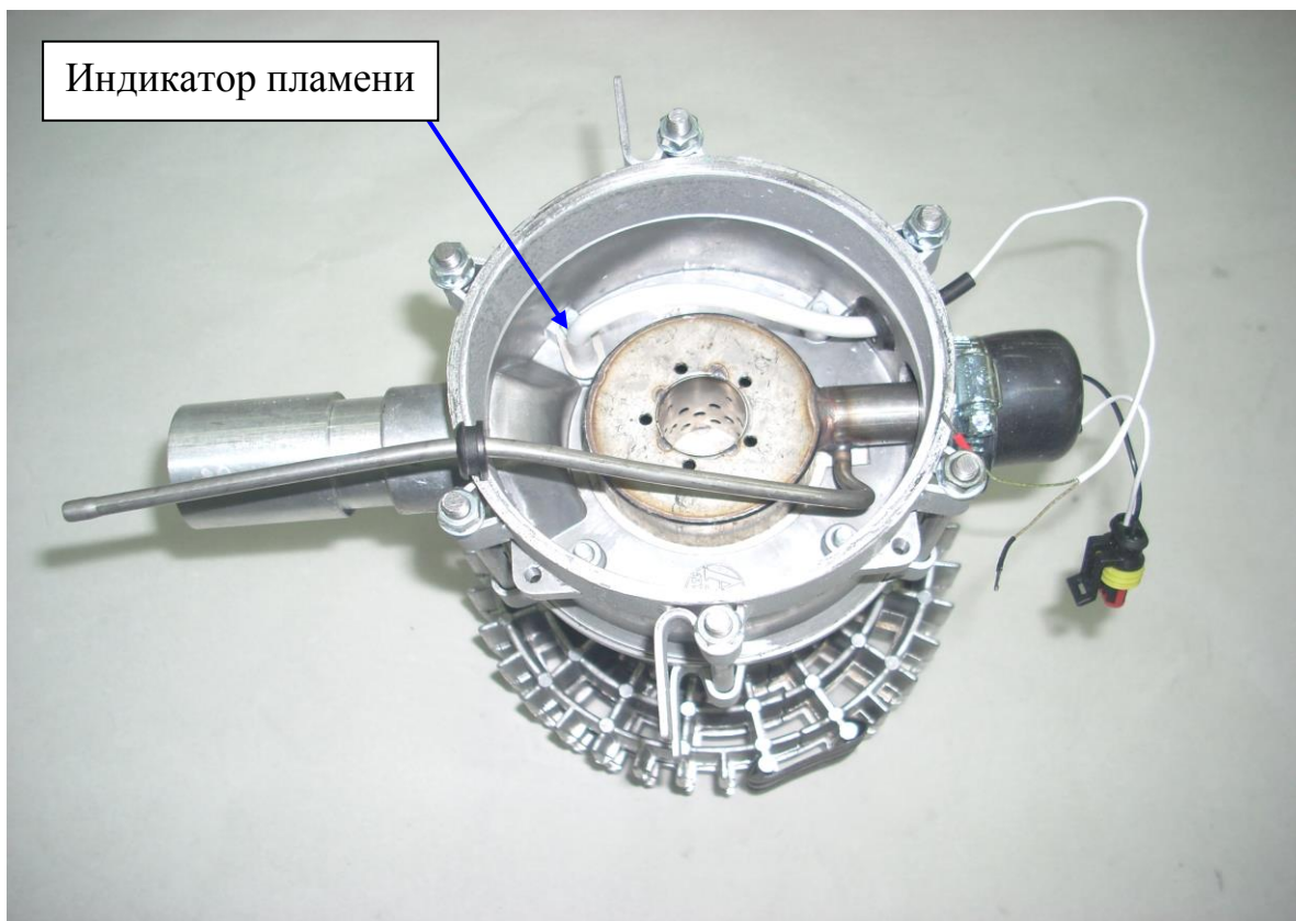
Рис.4 – Индикатор пламени.
